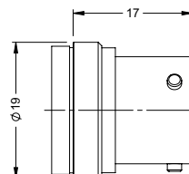
CONNETTORE A BAIONETTA MIL-C-26482 PER TEMPERATURA STANDARD (TB)
